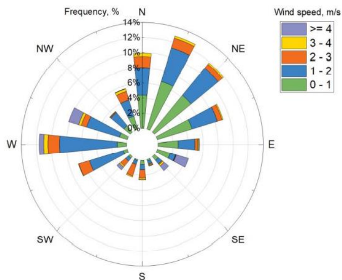
2 pav. Vėjo greitis ir kryptys
