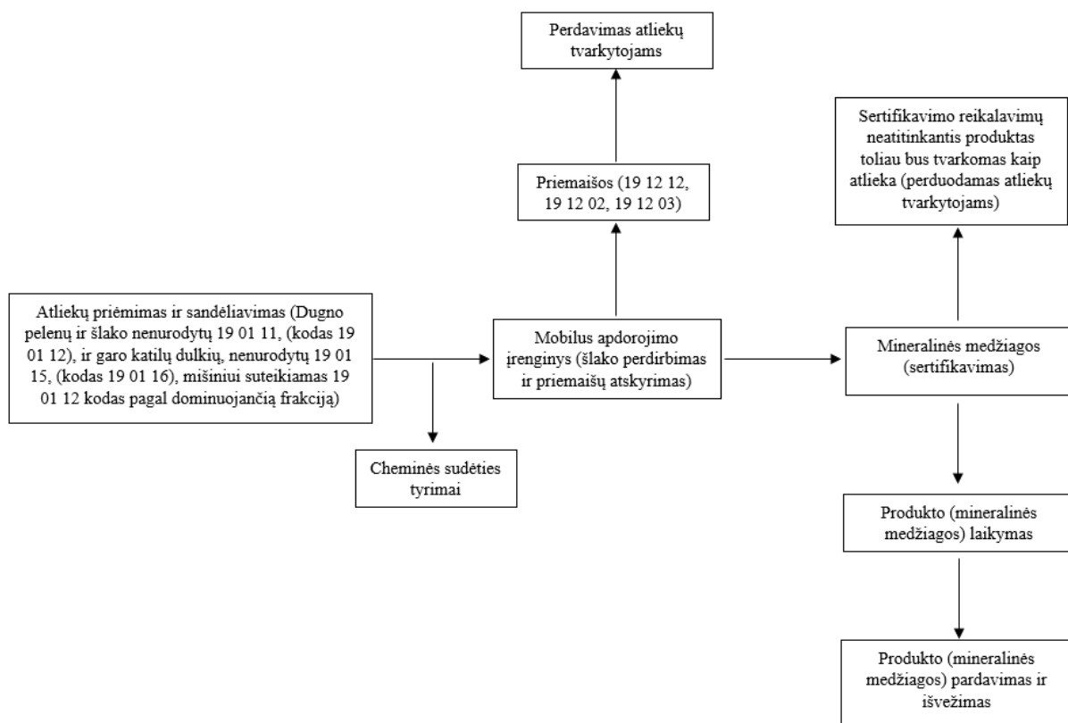
1.2.9.11 pav. Atliekų 19 01 12 principinė tvarkymo schema
