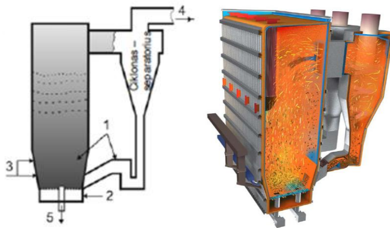
1.2.9.8 pav. Principinė cirkuliacinio verdančio sluoksnio pakuros schema: 1 – inertinis sluoksnis; 2 – pirminis oras; 3 – antrinis oras; 4 – degimo produktai; 5 – dugno pelenai.
