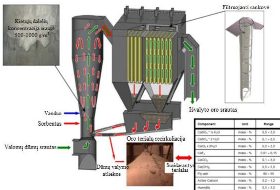
1.2.9.6 pav. Dūmų valymo sistema
