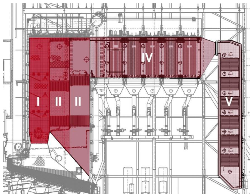
1.2.9.3 pav. Mišraus tipo atliekų garo katilas
